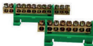
BORNIER DE REPARTITION SUR SUPPORT TS-0609F 6x9 8 poles 12 poles
